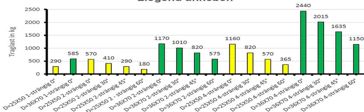
Chart 3: Winkel zwischen Muffenachse und Faserrichtung 90°
